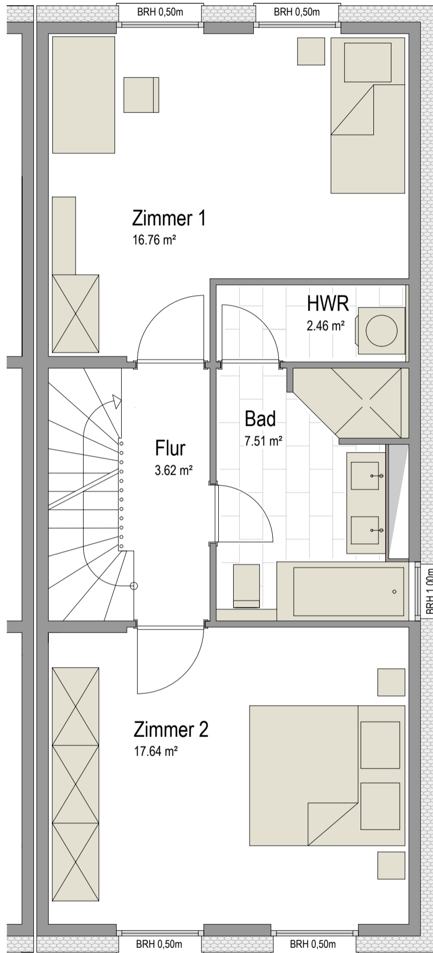
1.OBERGESCHOSS
